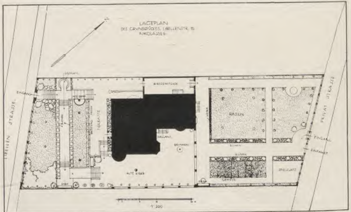
ARCH. ALFRED GREXANDER, BERLIN • HAUS BOUSSET IN NIKOLASSEE BEI BERLIN: GARTENSEITE UND LAGEPLAN
