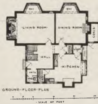
ARCH. TIMOTHY HONNOR • GRUNDRISS ZUM LANDHAUS IN GREAT MISSENDEN (VGL. SEITE 166)
