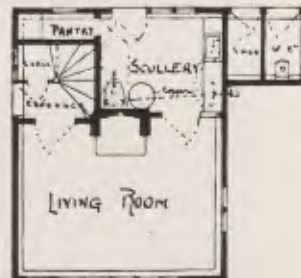
ARCH. OSWALD P. MILNE MODELL EINES SOMMERHÄUSCHENS (BACKSTEINBAU MIT RAUHEM BEWURF U. BRETTVERSCHALUNG) (BAUKOSTEN 3000 Mk.) ●●●●●
