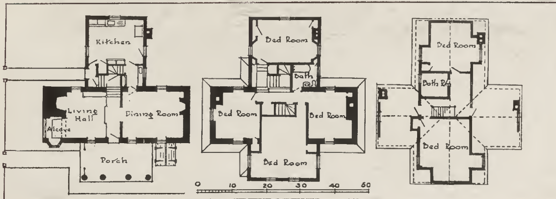
GRUNDRISSE EINES KLEINEN AMERIKANISCHEN LANDHÄUSCHENS
