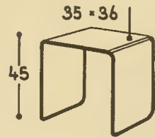
B 9s THONET Entwurf M. Breuer
