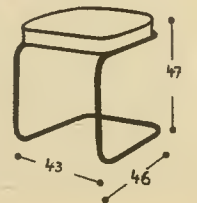
FH 58 P THONET Internationales künstlerisches Urheberrecht Entwurf M. Stam
