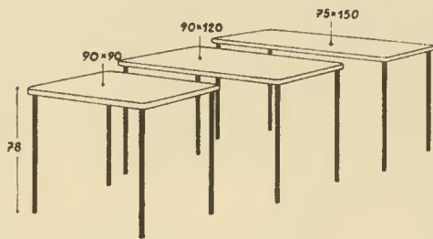
B 14/1 B 14/2 THONET Entwurf M. Breuer
