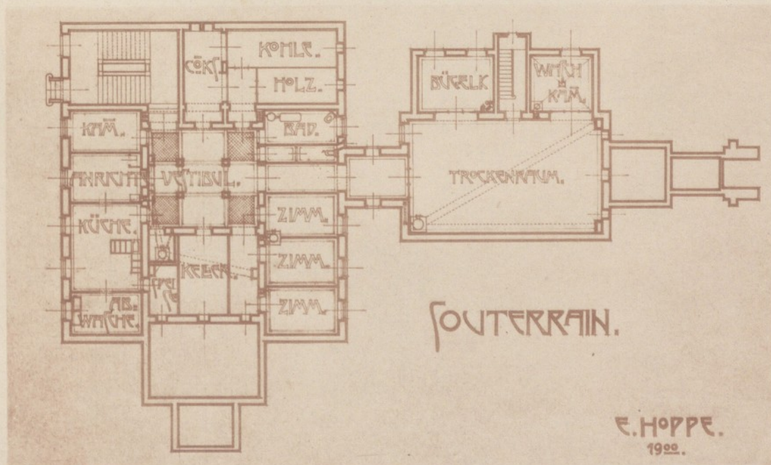
EMIL HOPPE. ENT- WURF FÜR EIN KÜNSTLERHEIM.
