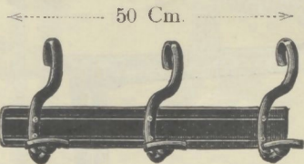
Kleiderrechen Nr. 5 mit 3 Bügelhaken K 4.— Nr. 11.135 " 4 " " 5.— " 11.145
