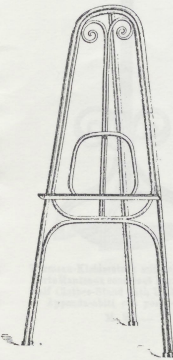
Maler-Staffelei Chevalet. Painters Easel. Cavalletto da disegno. Nr. 1. M. 36. —
