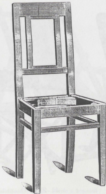
N. 22 - Da imbottire sedile cm. 42 x 40 altezza .. 93
