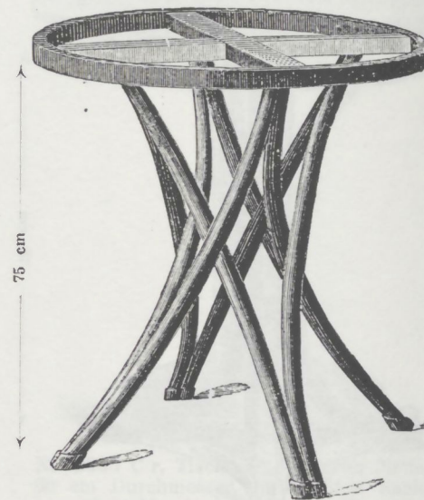
Nr. 8914, Tischgestell für Platten von 70—80 cm Durchmesser M. 16.—
