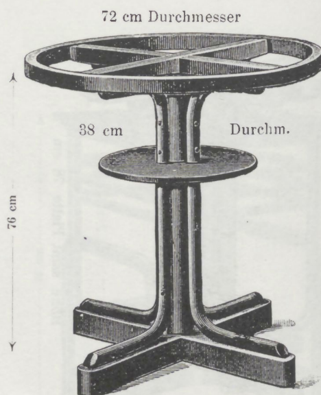
Nr. 8249, Tischgestell mit Fachplatte für Platten von 80 cm Durchmesser mit Zarge . . . . . M. 19.— Nr. 8449, ohne Zarge . . . . . „ 16.—
