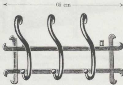
Nr. 11031 K, Kleiderrechen mit 3 Haken mit Kugeln M. 5.80 " 11041 K, " " 4 " " " 6.90 " 11051 K, " " 5 " " " 8.—
