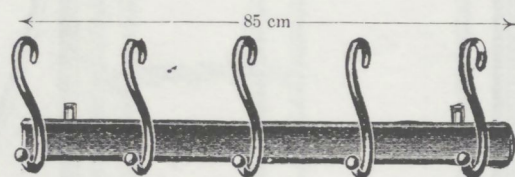
Nr. 11032 K, Kleiderrechen mit 3 Haken mit Kugeln M. 4.30 " 11042 K, " " 4 " " " 5.40 " 11052 K, " " 5 " " " 6.50
