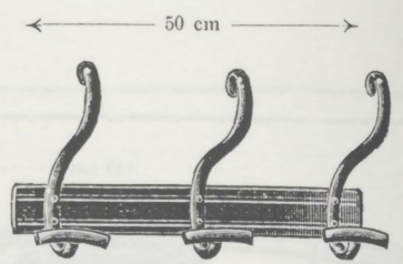
Nr. 11136, Kleiderrechen mit 3 Bügelhaken M. 4.20 " 11146, " " 4 " " " 5.30 " 11156, " " 5 " " " 6.40
