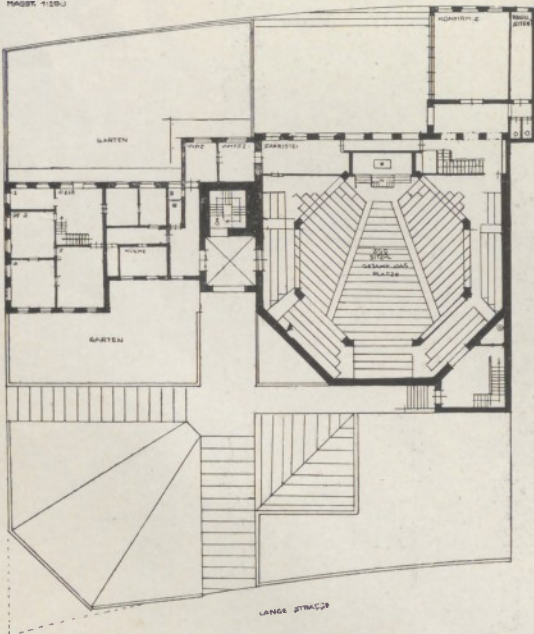
ERDGESCHOSS - GRUNDRISS MÄSSSTAB 1:200
