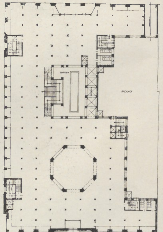
GRUNDRISS VOM ERDGESCHOSS MASSTAB 1:200
