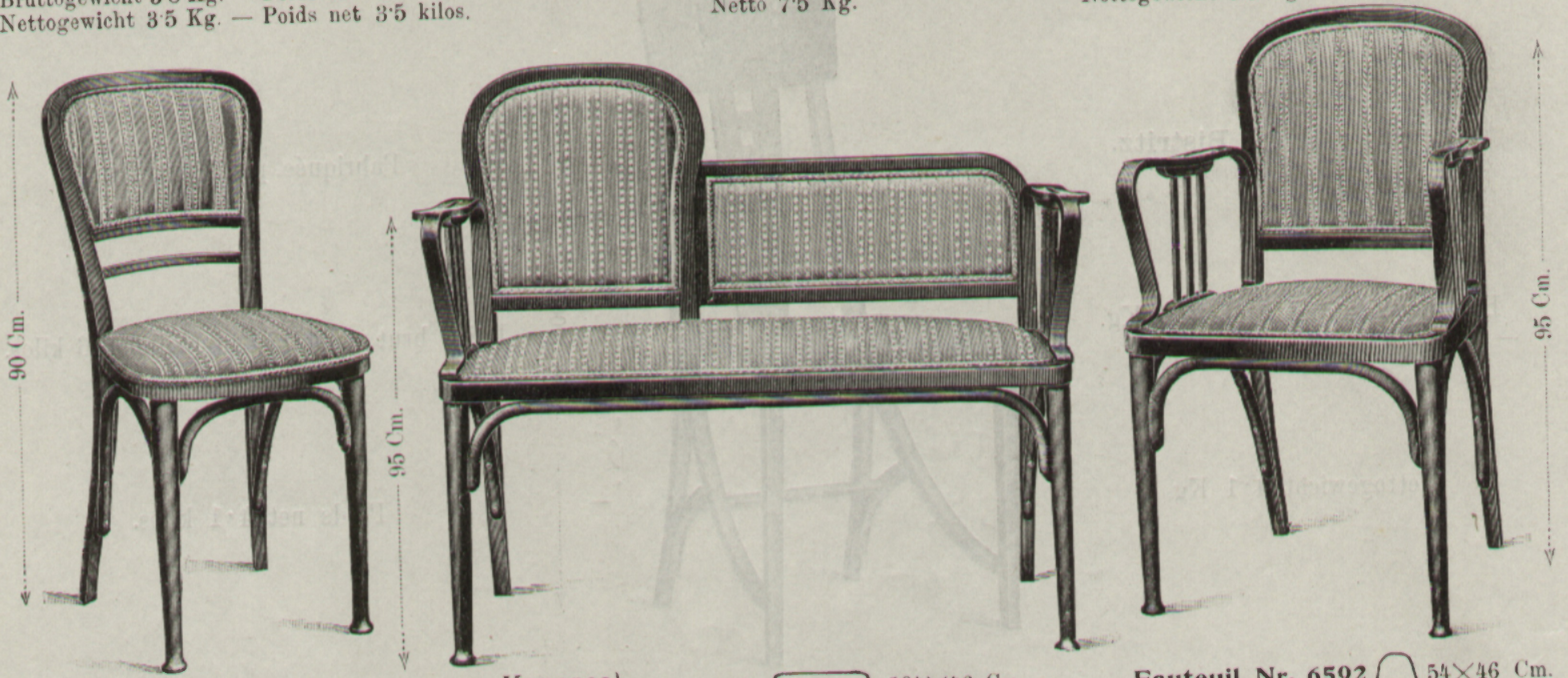
Sessel } Nr. 492 V 41 × 41 Cm. Kanapee } Nr. 6292 104 × 46 Cm. Fauteuil Nr. 6592 54 × 46 Cm. Chaise } Sitz grob vorgeflochten zum Polstern } a nicht geflochten zum Polstern } b Siège avec gros cannage à garnir } a non canné à garnir } b
